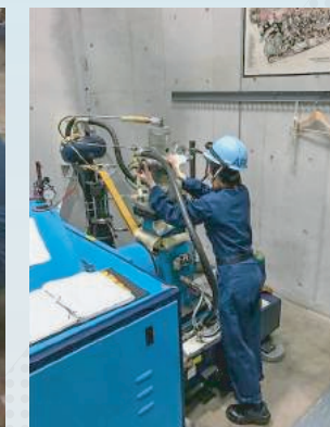
Adjust of the Injection pump 燃料ポンプの調整
